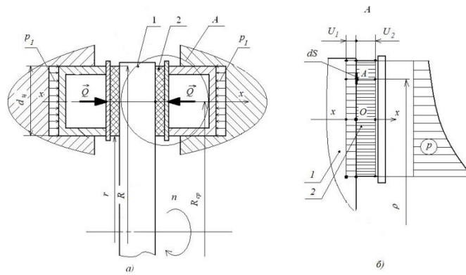
Рисунок 1 – Схема для визначення зносу дискового гальмівного механізму
