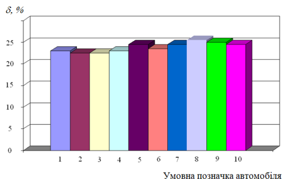
Рисунок 3 – Діаграма відносного зносу спряжених поверхонь тертя дискових гальмівних механізмів автомобілів
