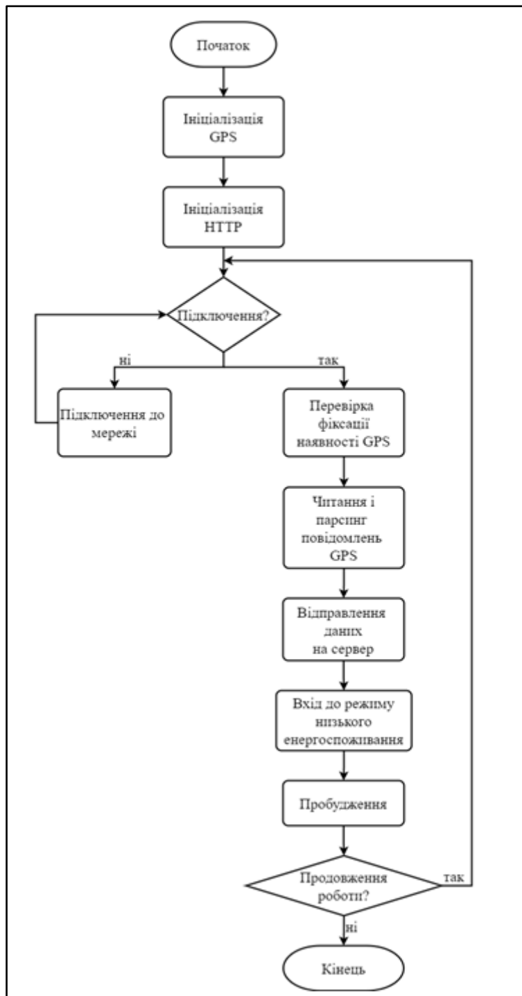
Рис. 2. Схема роботи GPS-трекера
